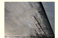
<床版鉄筋露出> 国道大和郡山上三橋線(極楽橋)
